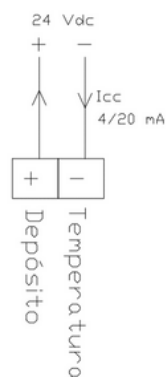
Sonda medida temperatura
