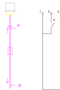
Ejemplo Sonda Nivel Contactos Digitales C2
